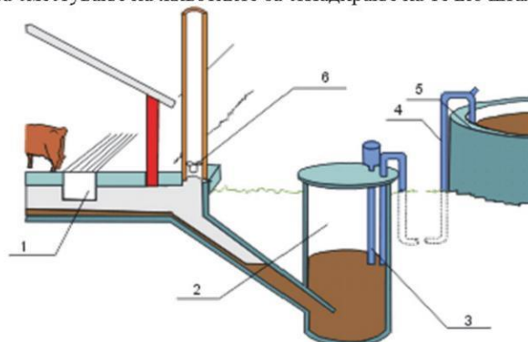
Систем за отстранување на течно ѓубре: 1 – канал за течно ѓубре; 2 - јама за препумпување; 3 - пумпа; 4 - нагорна цевка за течно ѓубре; 5 - резервоар за течно ѓубре; 6 – вентилатор
